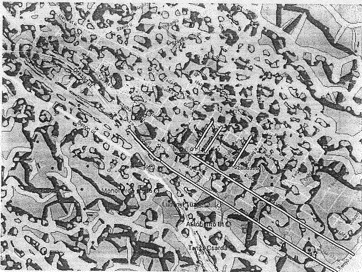
3. ábra. Domborzatból készített ú.n. "pocsolyatérkép". A világoskék-sötétkék foltok lefolyástalan, vagy helyi mélyvonulatban elhelyezkedő területek.
