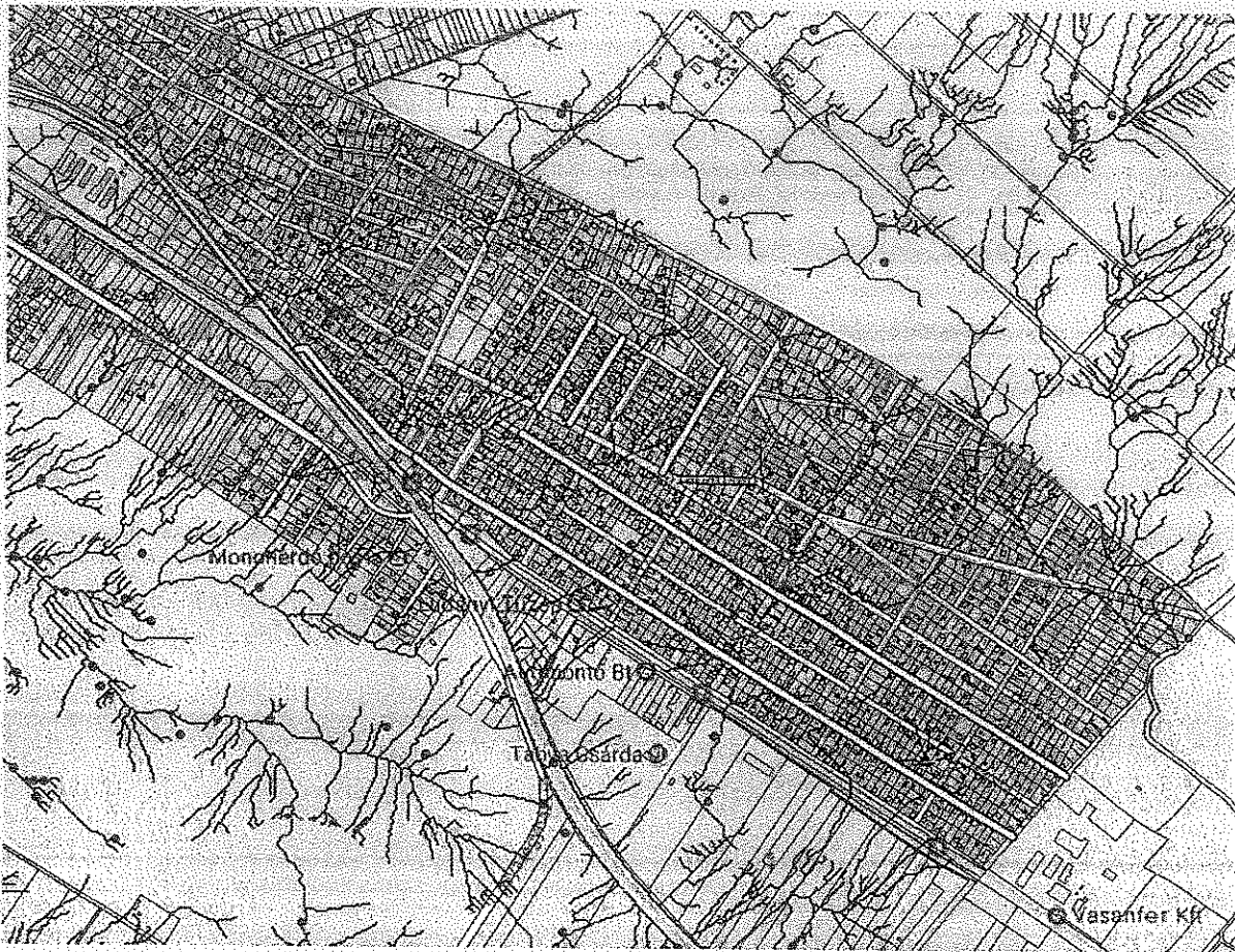
1. ábra. Településen domborzati viszonyok szerint kialakuló terepi lefolyási utak.
